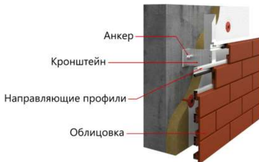
Рисунок 1. Конструктивная схема навесной фасадной системы с указанием основных элементов крепления [материал автора]
