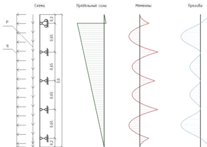
Рисунок 6. Расчетная схема и эпюры усилий, моментов и прогибов профиля для 2 варианта [материал автора]
