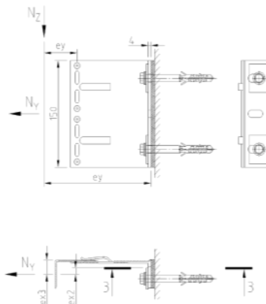
Рисунок 2. Схема крепления фасадного кронштейна(180 L+), к несущей стене и направления действующих нагрузок, используемые при выполнении расчётов [материал автора]
