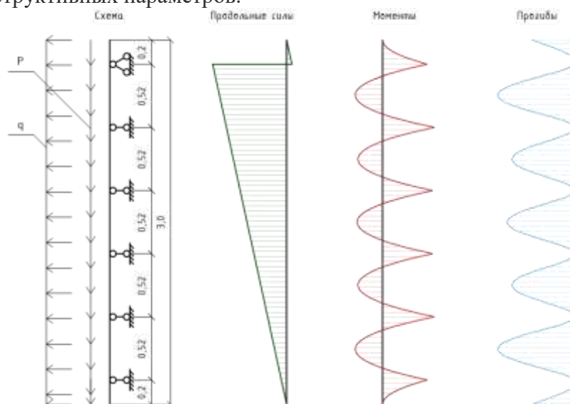
Рисунок 7. Расчетная схема и эпюры усилий, моментов и прогибов профиля для 3 варианта [материал автора]
