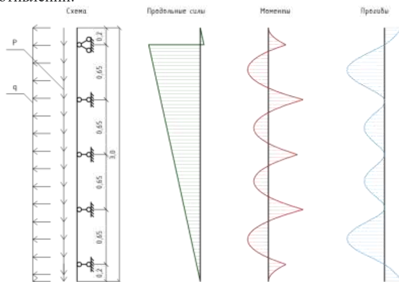
Рисунок 5. Расчетная схема и эпюры усилий, моментов и прогибов профиля для 1 варианта [материал автора]
