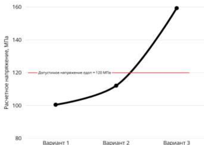
Рисунок 8. Сравнение напряжений в опорных кронштейнах для рассматриваемых вариантов подсистемы [материал автора]
