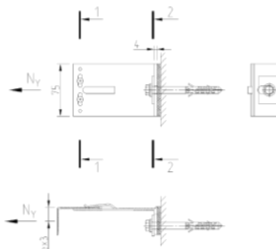
Рисунок 4. Схема крепления фасадного кронштейна (180 М), к несущей стене и направления действующих нагрузок, используемые при выполнении расчётов [материал автора]
