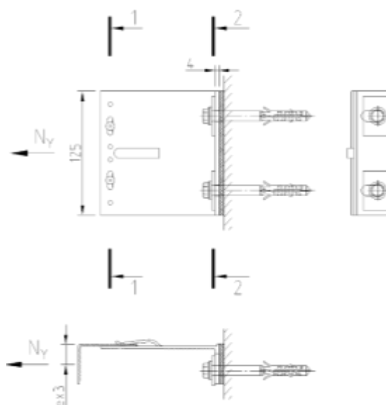
Рисунок 3. Схема крепления фасадного кронштейна(180 L), к несущей стене и направления действующих нагрузок, используемые при выполнении расчётов [материал автора]
